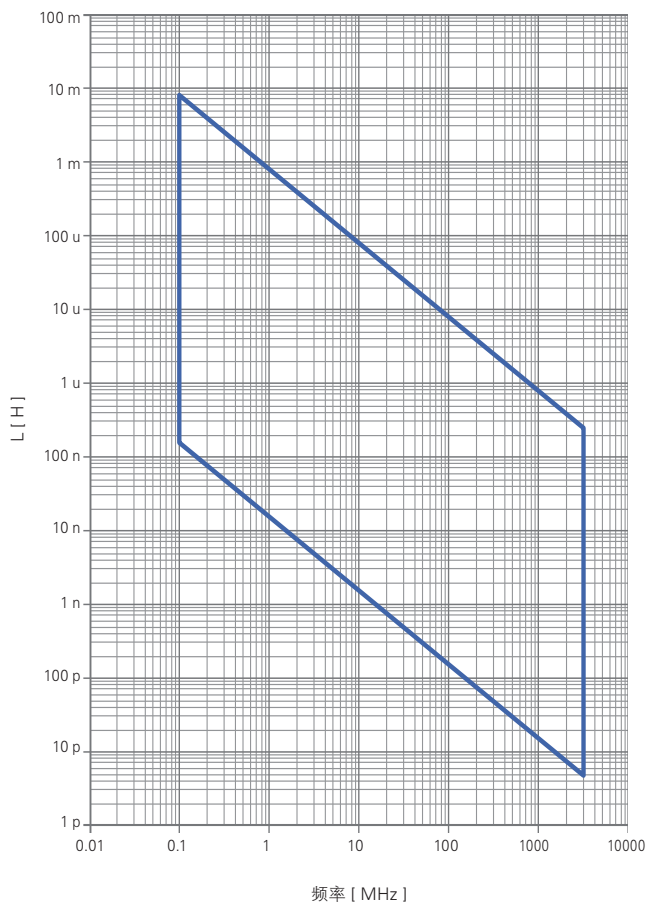
L 可测量范围
