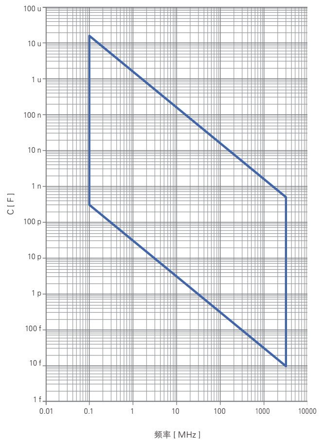
C 可测量范围
