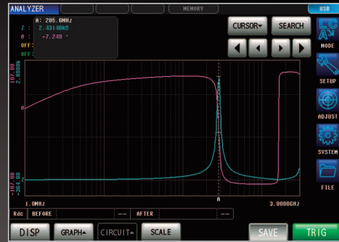
可稳定测量高达 3GHz 的阻抗
